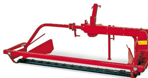
Balkenmähwerk Frontanbau
