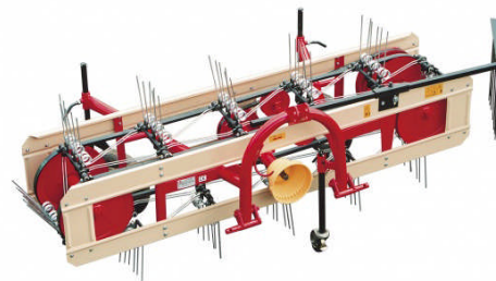
Sammelrechenmaschine
